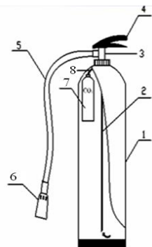
Bình bột chữa cháy MF
